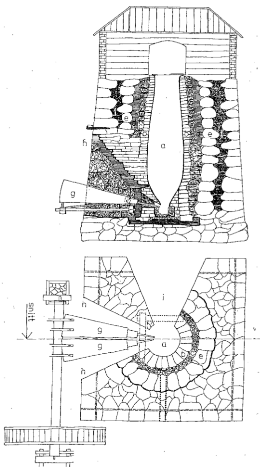
Figur 1: Masovn av vallonsk type med pipe (a) lagd av ildfast stein (b) omgitt av bakmur (c). Deretter sandfylling (d), ringmur e og fylling og yttermur av gråstein og leire (f). Kilde: Historisk leksikon.
