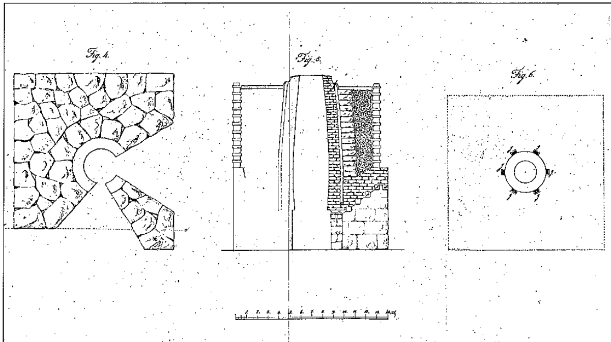
Figur 3: Tegningen fra 1799 viser rester av masovnen som var ved Verkensfossen på Bergs side. Ovnens var rast sammen til overstellet. Det er mulig å se en del av masovnpipa og noe av brystet ut mot elva. Råjernet ble tappet ut av et hull i den nederste del av pipa kalt stellet. Kilde: Johannessen 2000.
