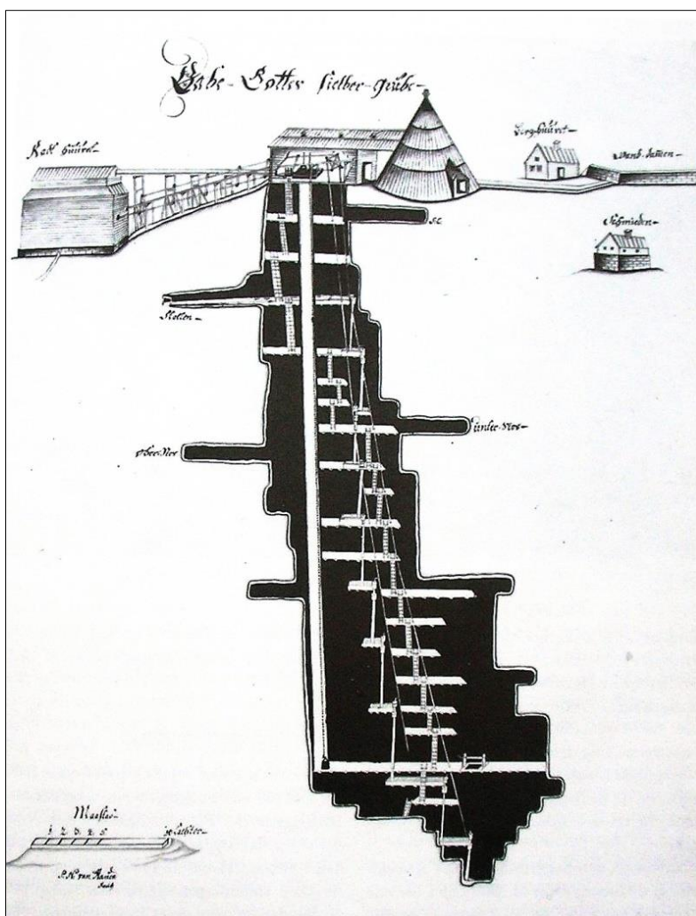
Snitt gjennom Gabe Gottes-gruva med stiger ned til gruvebunnen. Tegning fra 1700-tallet.
